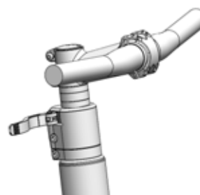
Illustration 115 : All Up avec levier de serrage de la potence ouvert
