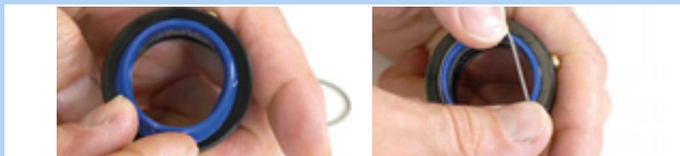
Illustration 184 : Insérer et fixer le joint anti-poussière
