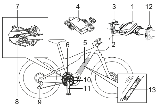
Illustration 25 : Schéma du système d'entraînement électrique
