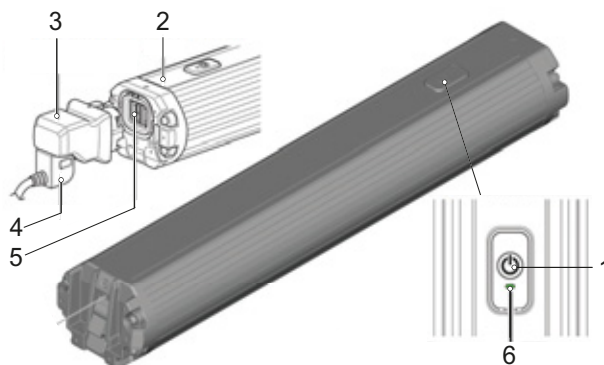
Illustration 26 : Vue d'ensemble de la batterie SHIMANO BT-E8036
