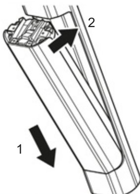
Illustration 104 : Insérer la batterie BT-E8036
