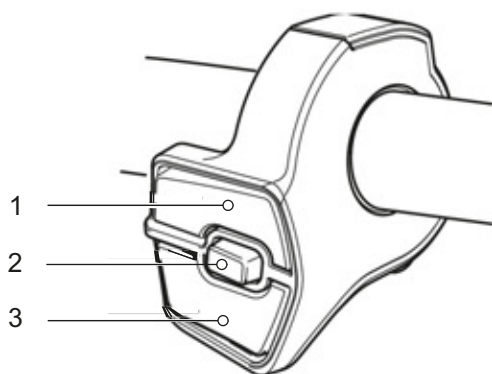
Illustration 31 : Unité de commande à 3 commutateurs
