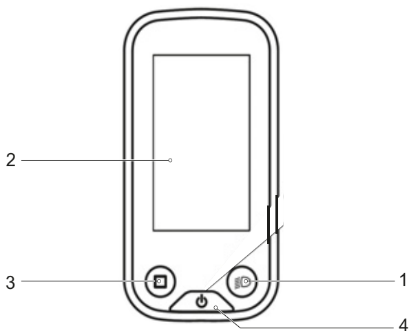
Afbeelding 29: Details boordcomputer SC-E6100
