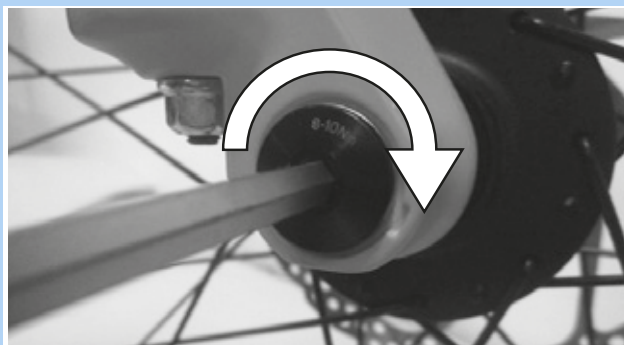
Afbeelding 42: As in de richting van de pijl vastdraaien
