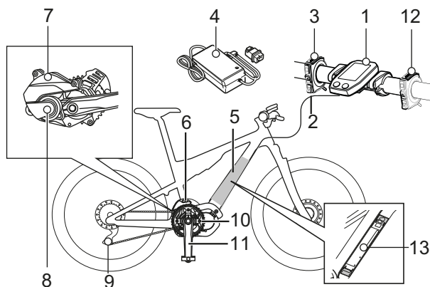
Afbeelding 25: Schema elektrisch aandrijfsysteem
