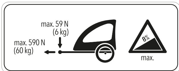
Afbeelding 96: Waarschuwingssticker aanhanger
