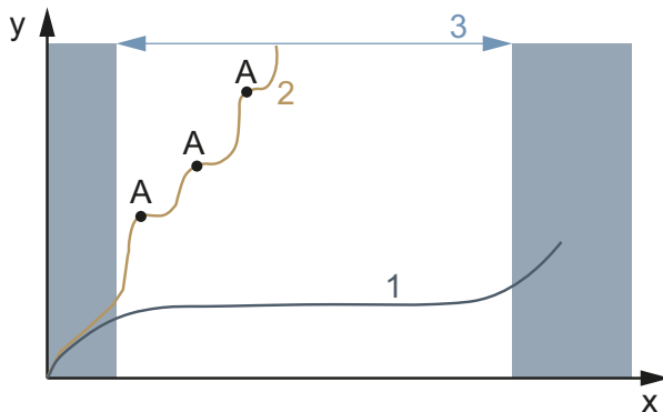
Afbeelding 121: Grafiek slijtage, bedrijfsduur (x) tegen materiaalaafname (y)
