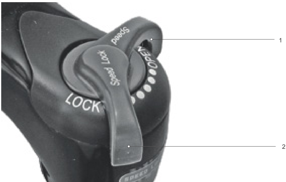
Afbeelding 116: Suntour drukdemper in open (1) en gesloten (2) stand
